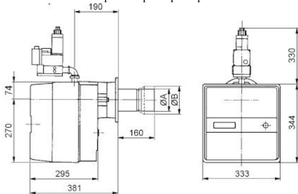
Габаритные размеры горелок
