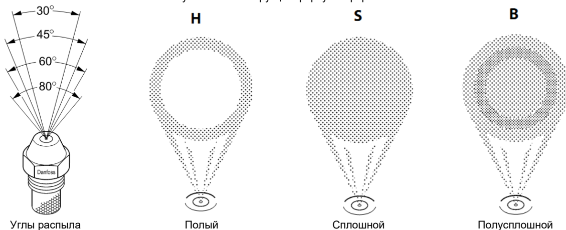
Рисунок 22 – Углы и рисунки распыла форсунок
