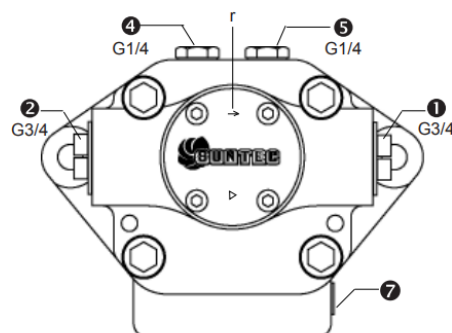
Насос шестеренчатый жидкотопливный марки Т Типоразмер 2-3-4-5
