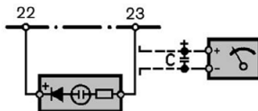
Микроамперметр (диапазон измерений 0...600 мкА или 0...1,0 мА)
