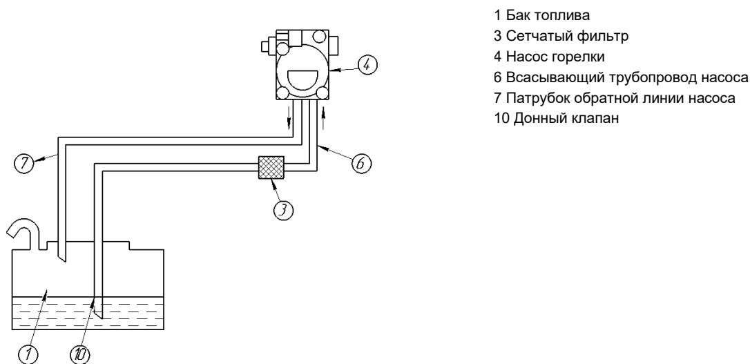
Рисунок 12 – Схема подключения горелки (насоса) по двухтрубной системе
