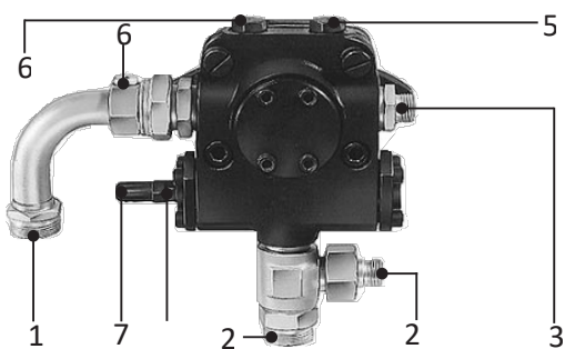
Насос шестеренчатый жидкотопливный марки ТА2
