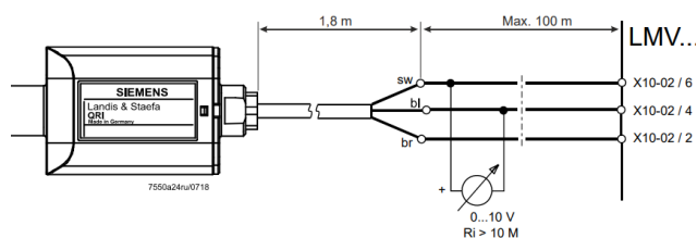
Вольтметр (диапазон измерений 0...30 В)
