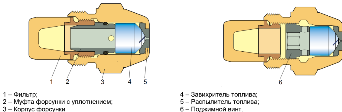
Рисунок 21 – Конструкция форсунки фирмы «Danfoss»
