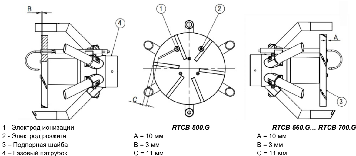
Рисунок 26 – Положение электродов горелок типа RTCB-500.GD... RTCB-700.GD
